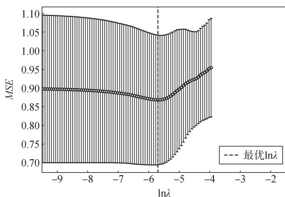
图 2 Lasso 交叉验证误差曲线
