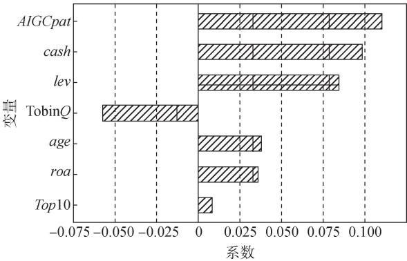
图 4 Lasso 回归变量系数
