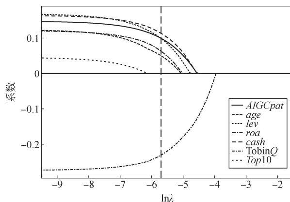
图 3 Lasso 系数路径
